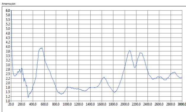
VSWR
