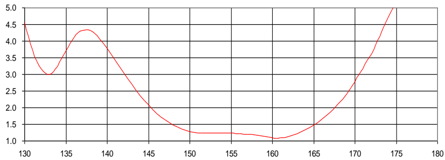
VSWR
