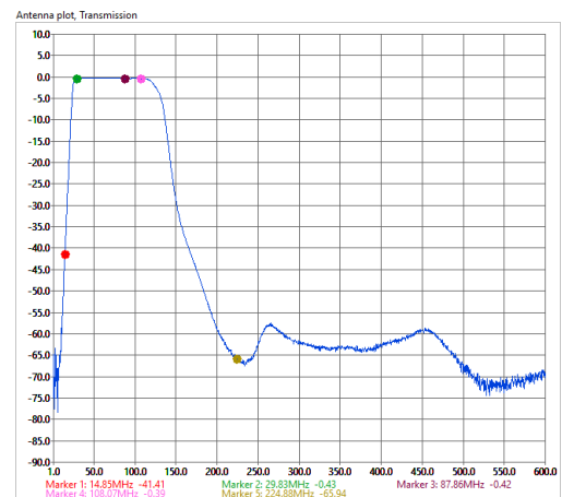
VHF 30-88 (108) MHz
