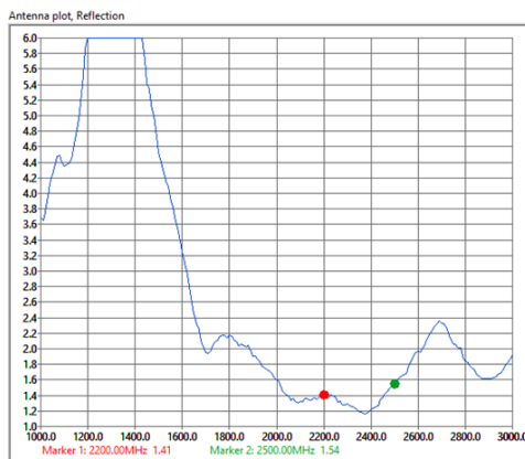
VSWR
